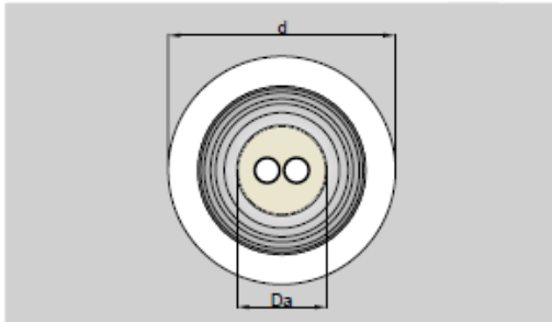
Abb. 39: Kernlochbohrung FibreFLEX/CaldoPEX double
